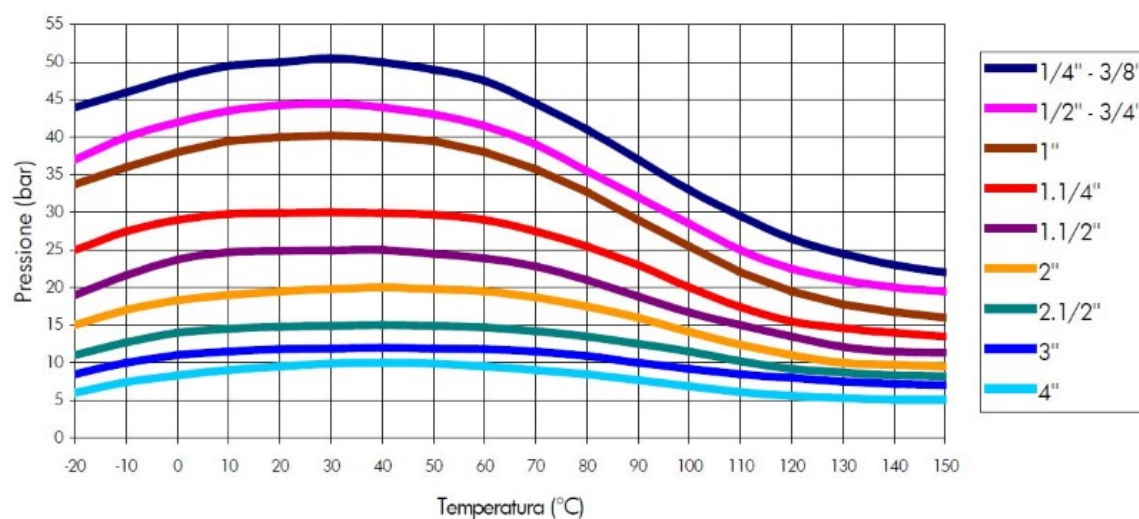
DIAGRAMMA PRESSIONE/TEMPERATURA
